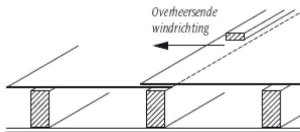
Verticale naden
