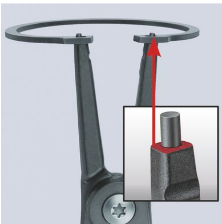
KNIPEX precisie borgveertang: makkelijke en snelle montage van de ring zonder verwringing
