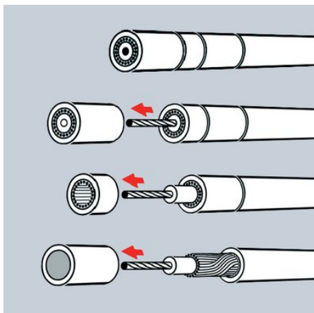
Driedelig afstrippen van een coax-kabel
