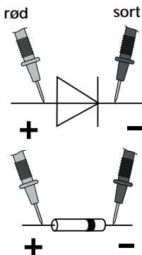
Gennemgangsretning
