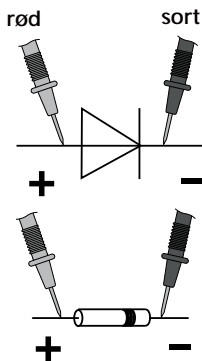
Gjennomgangsretning
