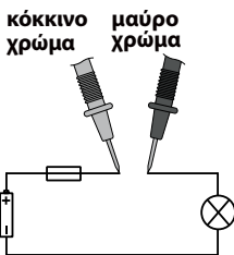
Κατεύθυνση διέλευσης
