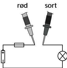
Gjennomgangsretning
