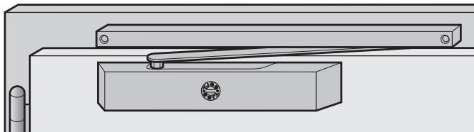
T46: Normale montage aan scharnierzijde
