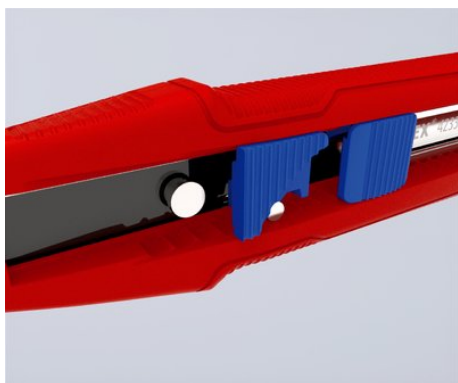
Trekvaste mesvergrendeling en mesborgpen van gehard staal
